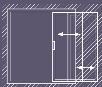
2 rails 2 vantaux
